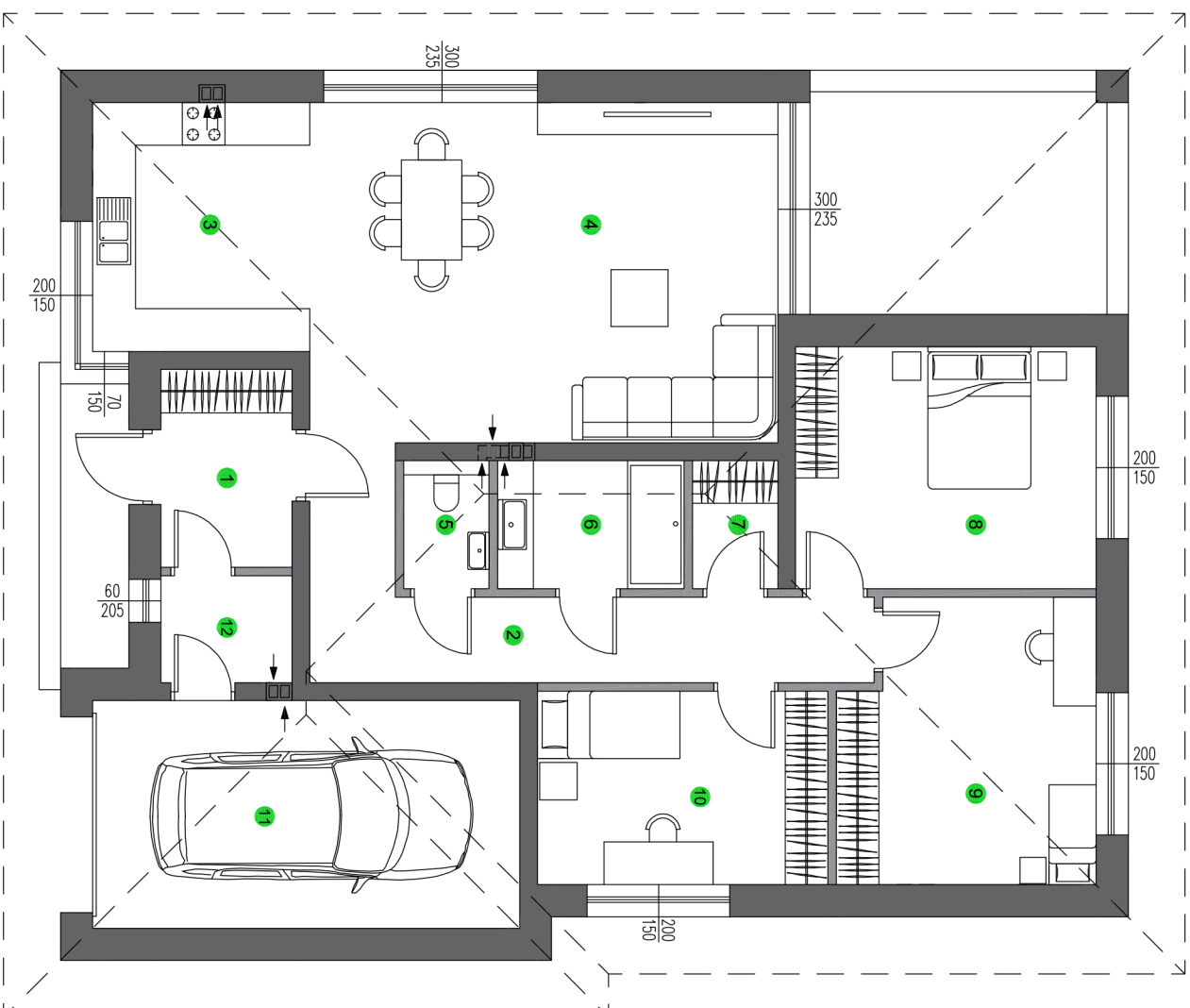
Rzut parteru
